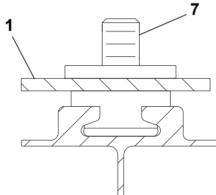
VIEW A-A
